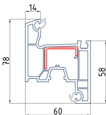
Створка 3-камерная 039
