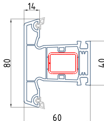
Импост 3-камерный 018
